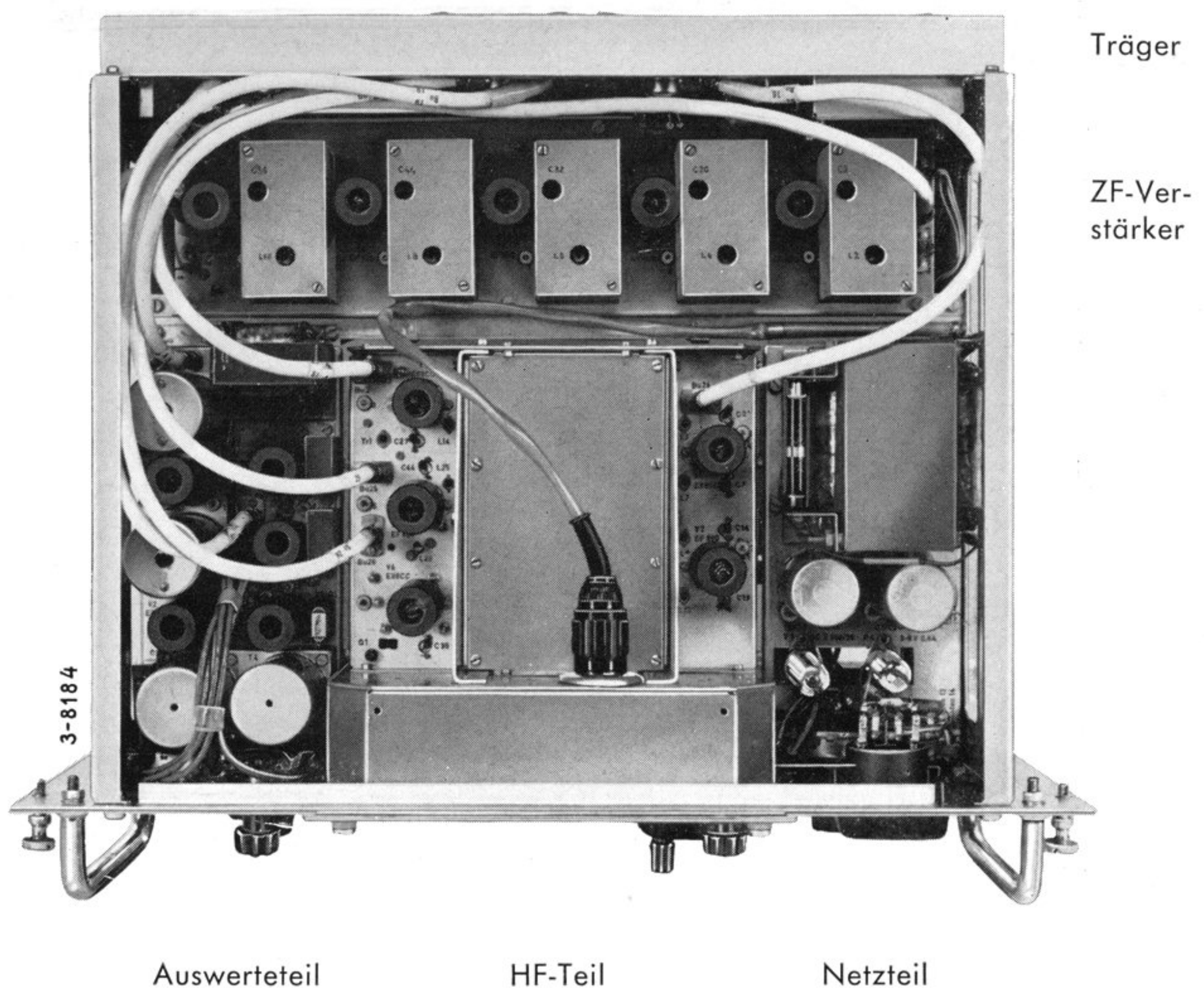
Bild 1 Ansicht des Empfängers von oben
