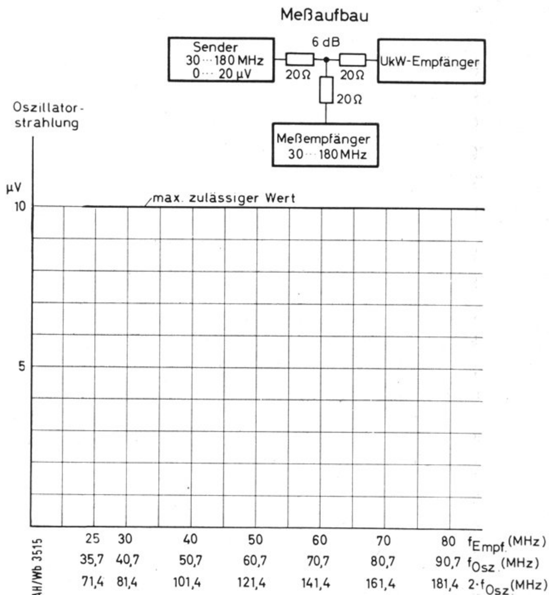
Bild 10 Messung der Oszillatorstrahlung
