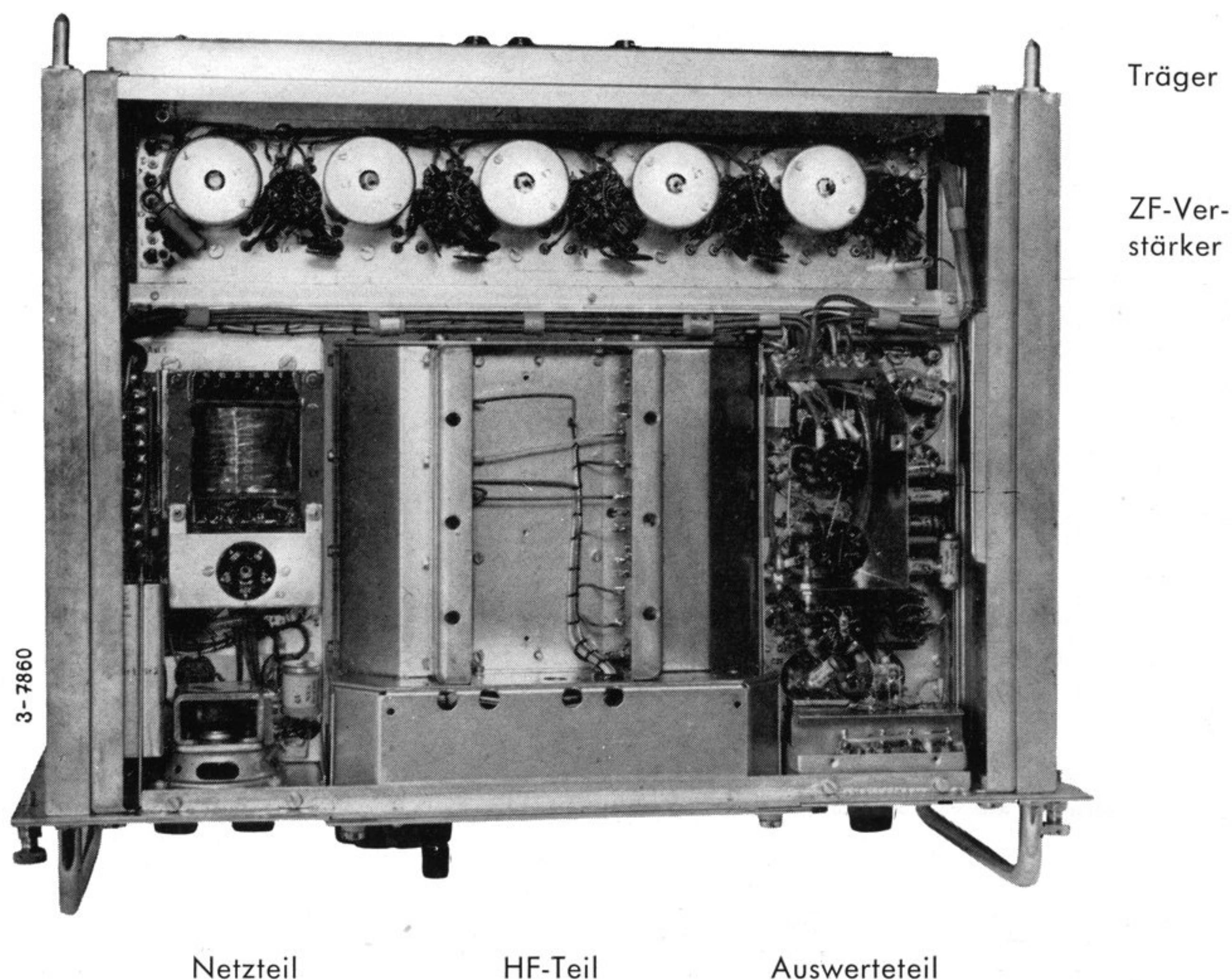
Bild 2 Ansicht des Empfängers von unten
