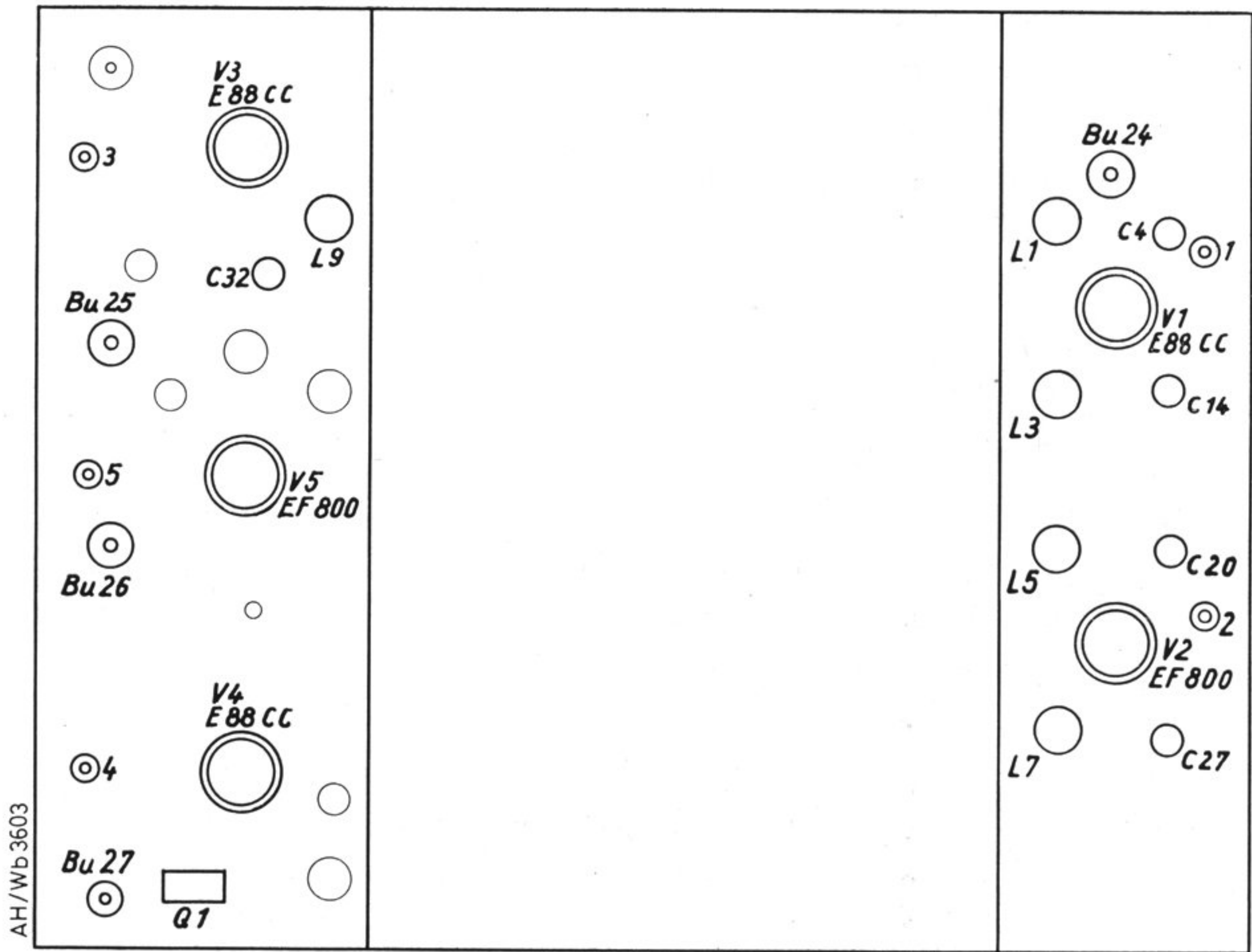
Bild 11 Meßpunkte am HF-Teil
