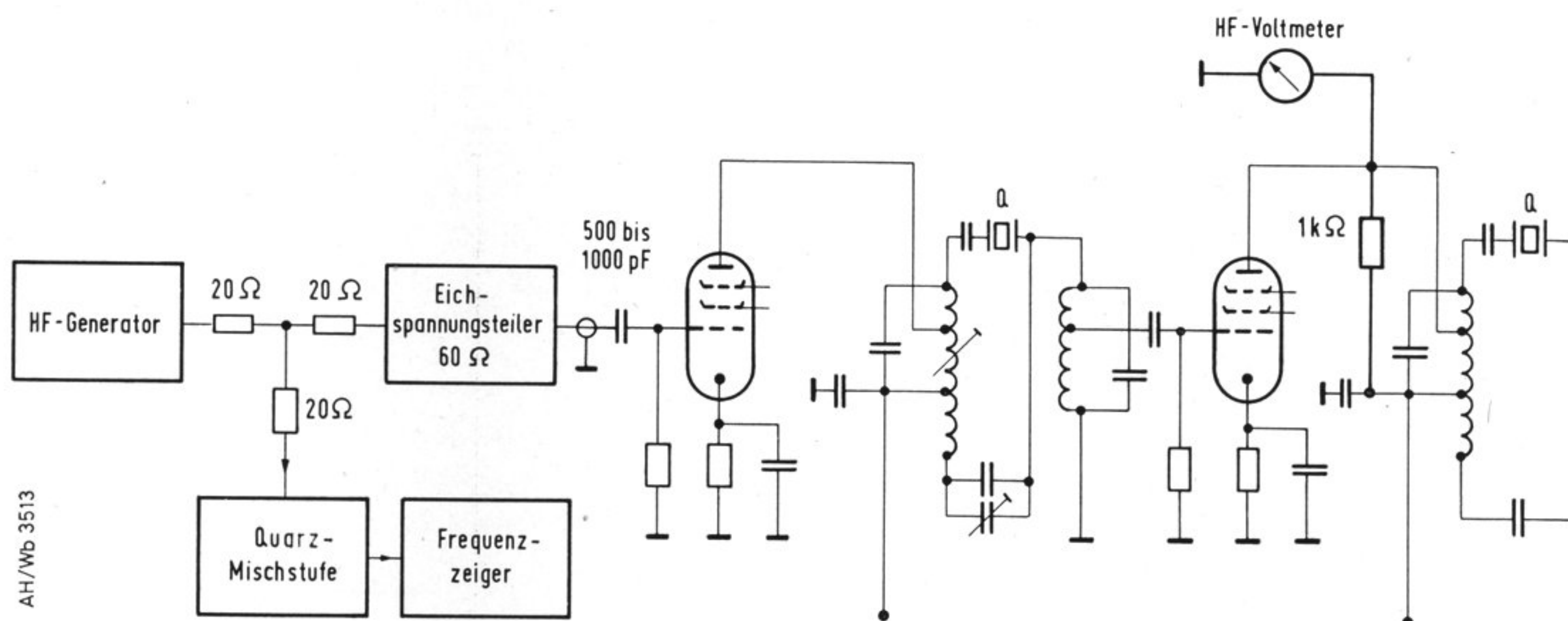
Bild 8 Meßaufbau
