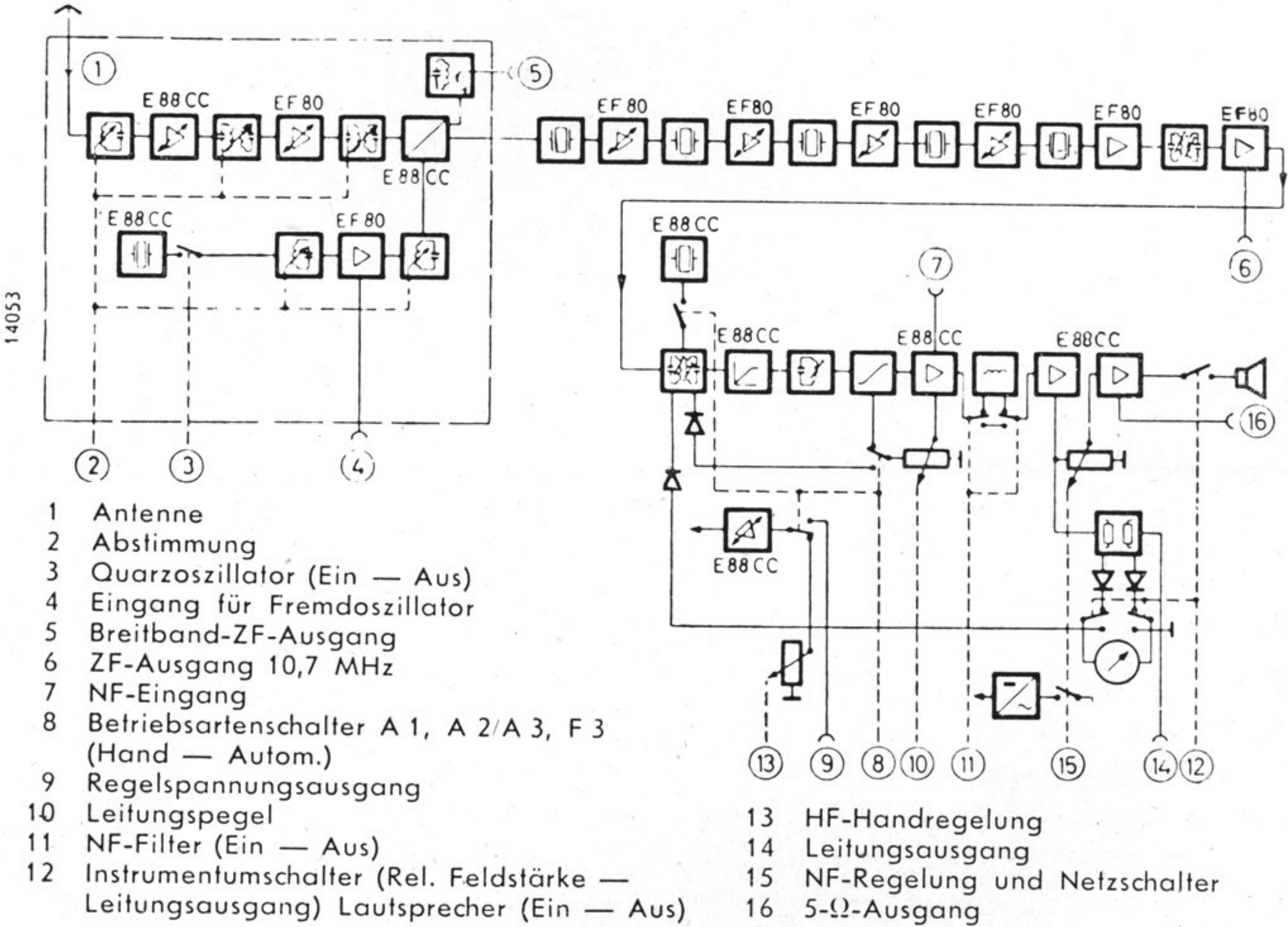
Bild 3 Übersichtsschaltplan
