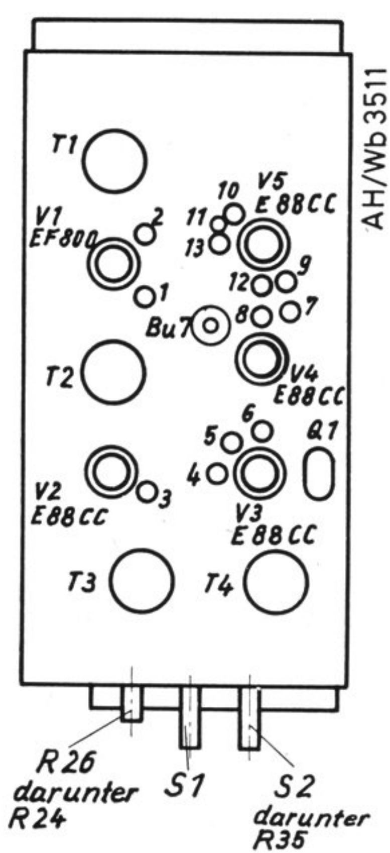
Bild 6 Meßpunkte am Auswerteteil
