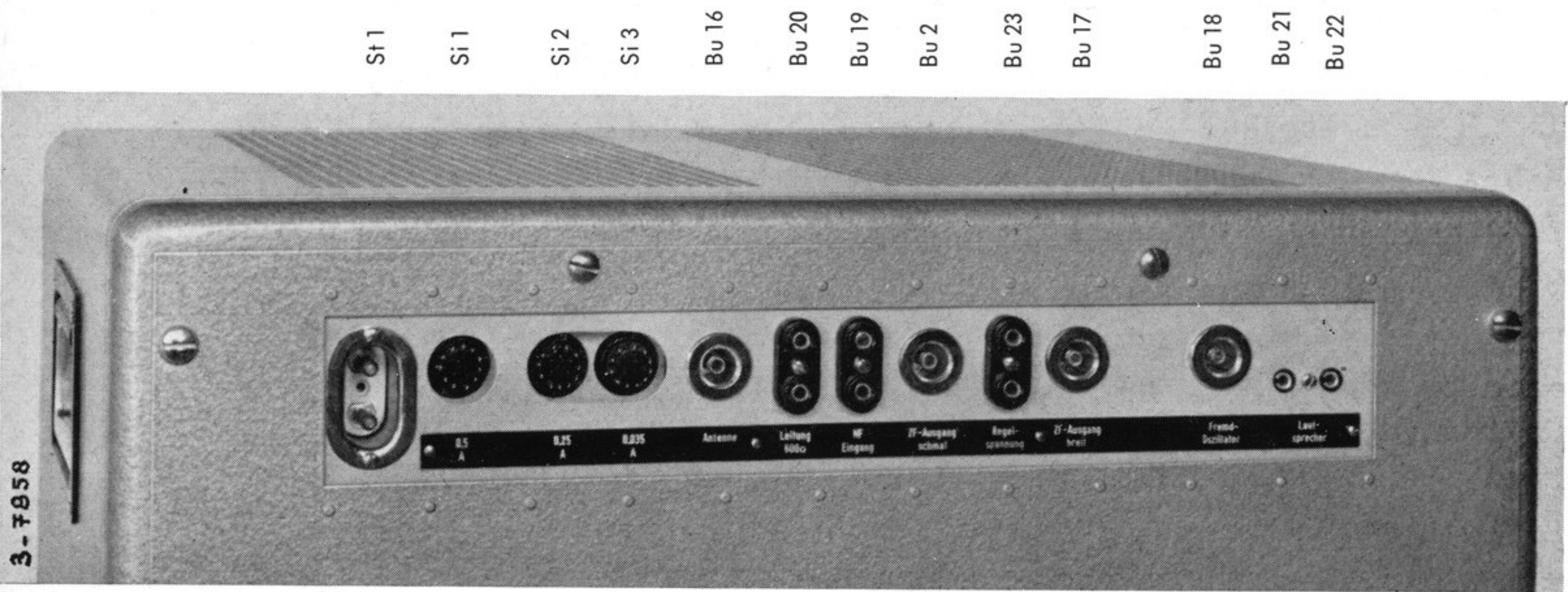
Bild 4 Rückwärtige Anschlüsse (und Sicherungen)
