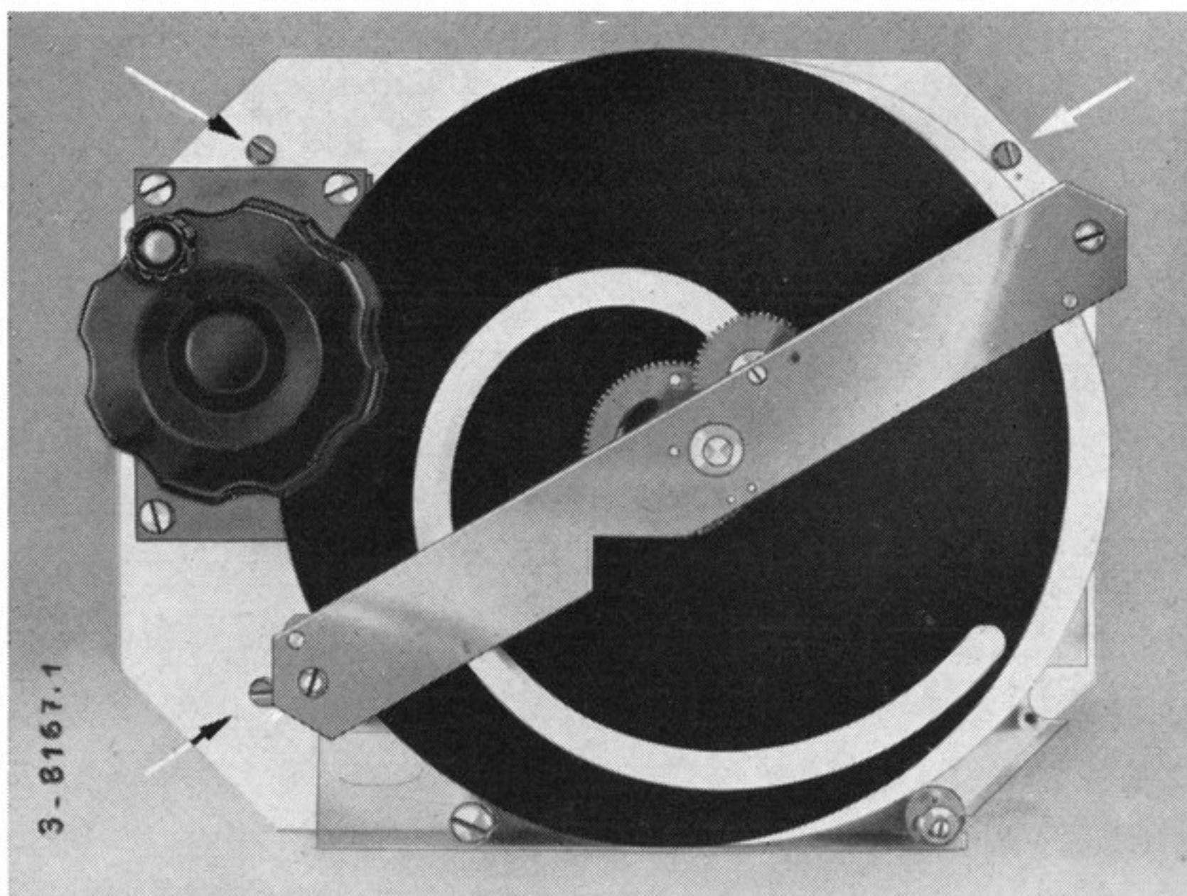
Bild 5 Frequenzeinstellknopf mit Skalenmechanismus (Pfeile bezeichnen die drei Befestigungsschrauben)
