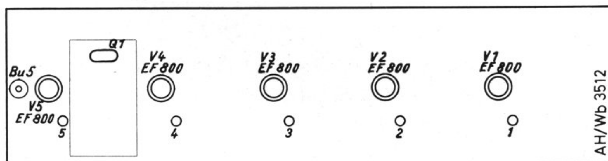
Bild 7 Meßpunkte an den Kathoden des ZF-Verstärkers
