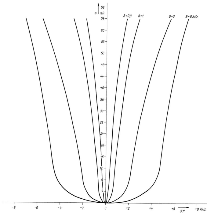
Bild 10 Gesamtselektion des Empfängers bei Zweiseitenband-Betrieb
