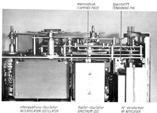
Bild 6 Getriebe von unten gesehen
