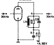
SINGLE CIRCUIT Einzelkreis
