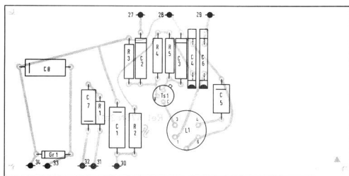
100-kHz-Raster Rel 455 N 300c1 (von rechts) mit Versorgungsplatte Rel 455 N 302a3 100-kHz SPECTRUM UNIT Type Rel 455 N 300c1 (FROM THE RIGHT) WITH SUPPLY BOARD Type Rel 455 N 302a3
