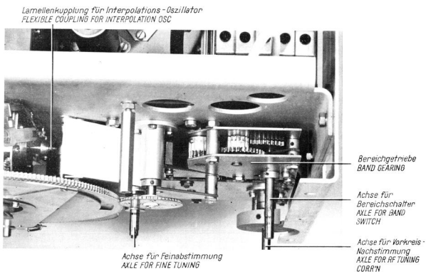
Bild 7 Bereichsgetriebe und Lamellenkupplung
